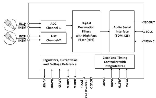
概略ブロック図
