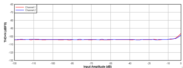
9-7. PCM1821-Q1: THD+N vs Input Amplitude
