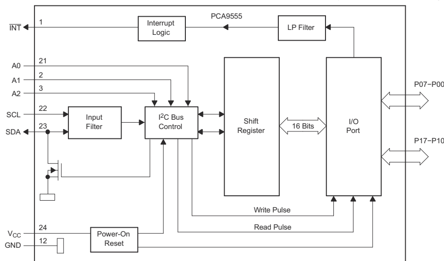
ブロック図
