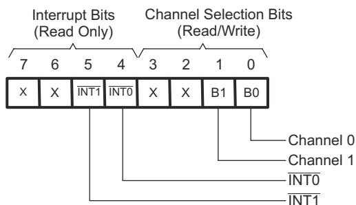
图 8-8. Control Register
