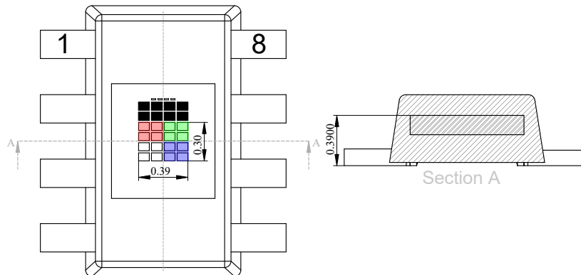
図 9-2. Sensor Position
