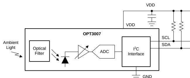
ブロック図
