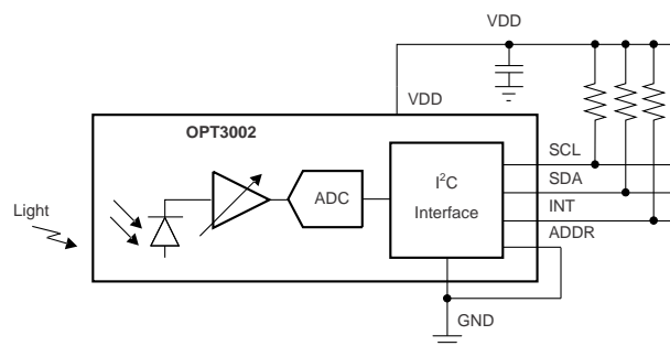
ブロック図
