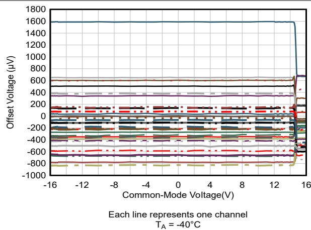
图 5-7. Offset Voltage vs Common-Mode Voltage
