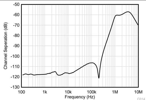
図 5-40. チャネル・セパレーションと周波数との関係
