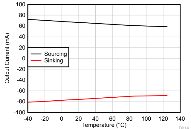
図 5-38. 短絡電流と温度との関係
