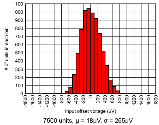
図 6-26. Input Offset Voltage Histogram
