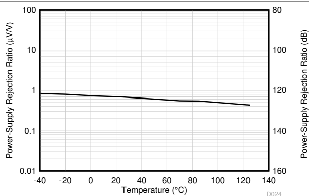
図 5-24. PSRR と温度との関係
