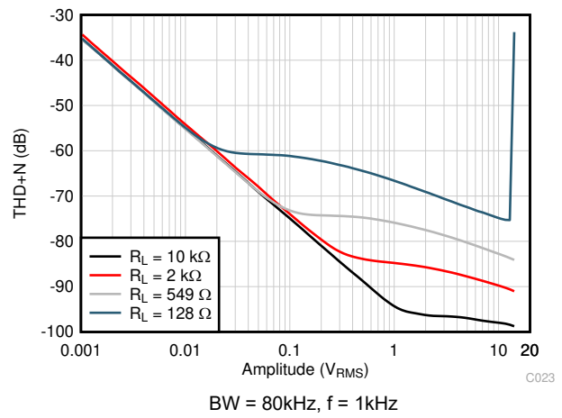
図 5-24. THD+N vs Output Amplitude
