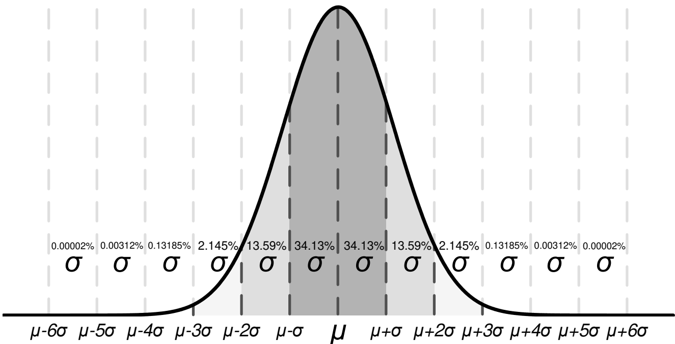
図 6-11. Gaussian Distribution
