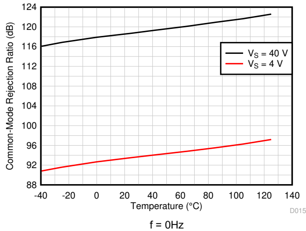
図 5-19. CMRR vs Temperature (dB)
