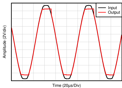
図 6-9. No Phase Reversal
