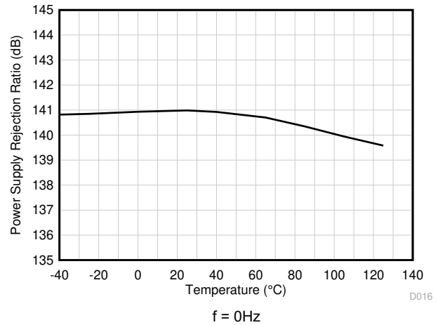
図 5-20. PSRR vs Temperature (dB)
