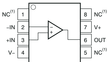
图 5-3. OPA376-Q1: D (8-Pin SOIC) Package, Top View
