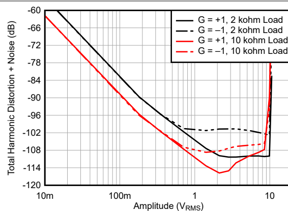
図 5-26. 全高調波歪 + ノイズ比と出力振幅との関係
