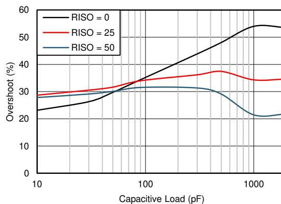
図 6-32. 小信号オーバーシュートと容量性負荷との関係 (出力ステップ 100\text{mV} )
