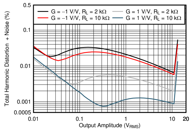
図 6-26. THD+N と出力振幅との関係
