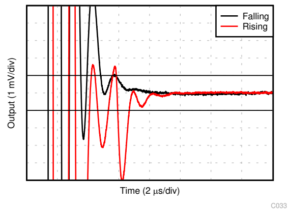
図 6-38. セトリング・タイム (1V 正ステップ)
