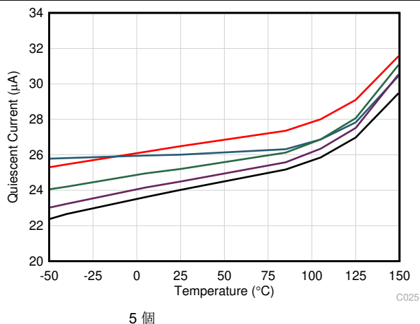
図 6-26. 静止電流と温度との関係
