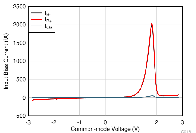
図 6-10. 入力バイアス電流と同相電圧との関係
