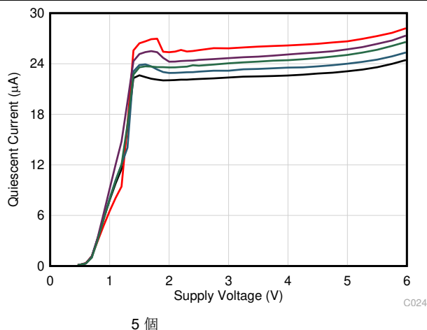
図 6-25. 静止電流と電源電圧との関係
