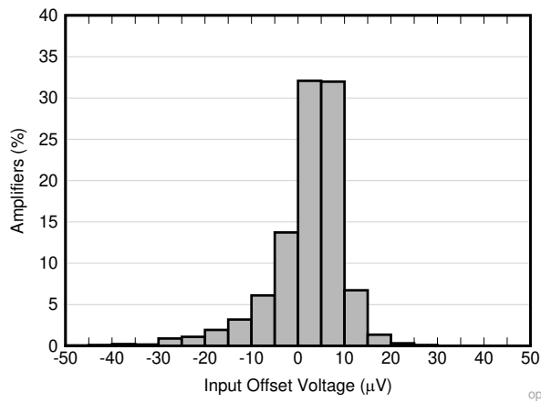
図 6-1. オフセット電圧の分布
