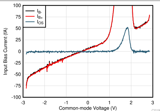
図 6-9. 入力バイアス電流と同相電圧との関係
