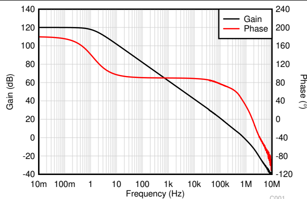
図 6-7. 開ループ・ゲインおよび位相と周波数との関係
