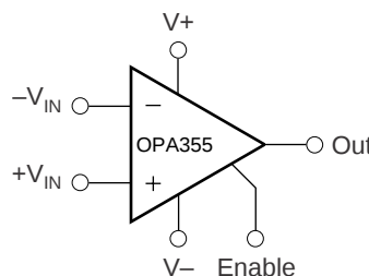
概略回路図
