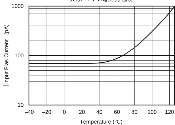
入力バイアス電流 対 温度
