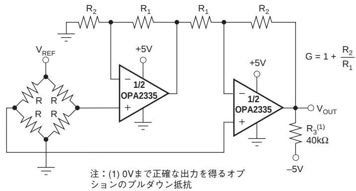
図6. デュアル・オペアンプによるIAブリッジ・アンプ
