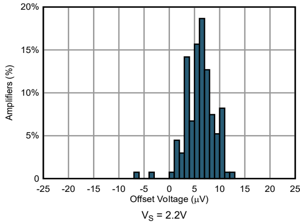
図 5-1. オフセット電圧の製品分布
