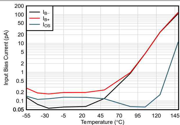
図 5-8. 入力バイアス電流と温度との関係
