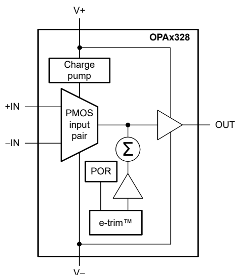
ブロック図
