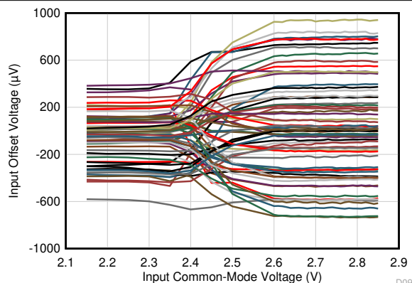
図 5-9. オフセット電圧と同相電圧との関係
