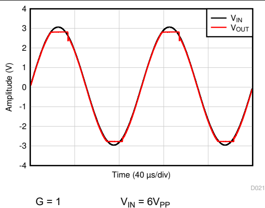
図 5-41. 位相反転が発生しない
