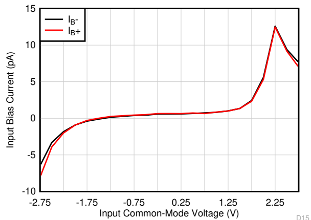
V_+ = 2.75\text{V} , V_- = -2.75\text{V} , V_{CM} = V_S/2 図 5-15. I_B と同相電圧との関係
