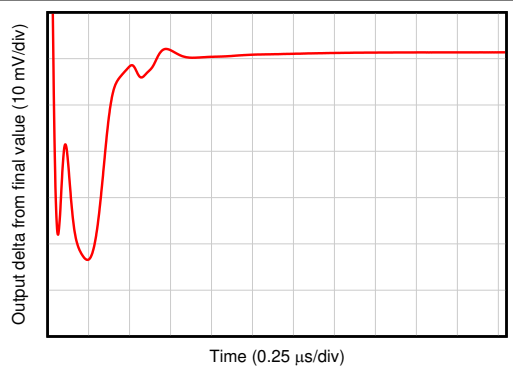
図 5-45. 小信号ステップ応答
