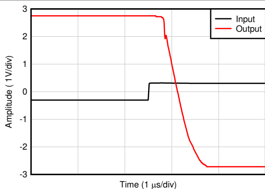
図 5-43. 過負荷回復
