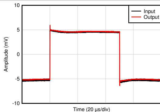
図 5-44. 小信号ステップ応答
