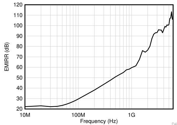
図 5-52. 非反転入力を基準とする電磁干渉除去比 (EMIRR+) と周波数との関係
