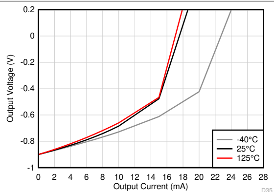
図 5-22. 出力電圧スイングと出力電流との関係 (シンク)
