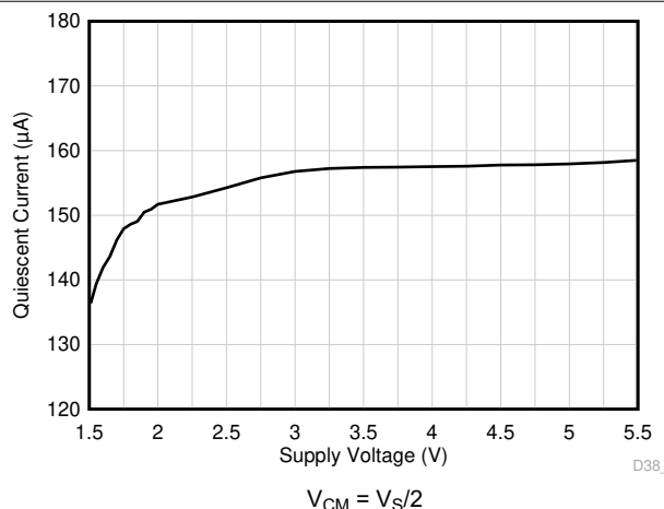
図 5-35. 静止電流と電源電圧との関係
