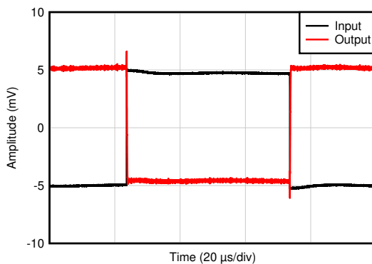
図 5-43. 過負荷回復
