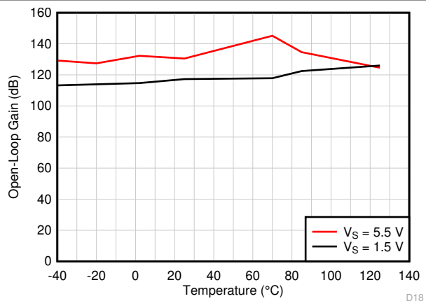
R_L = 10\text{k}\Omega 図 5-17. 開ループゲインと温度との関係
