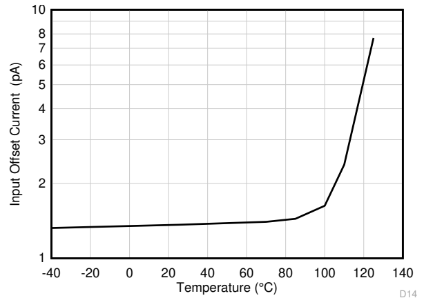
V_S = 5.5\text{V} , V_{CM} = V_S/2 図 5-14. I_{OS} vs 温度
