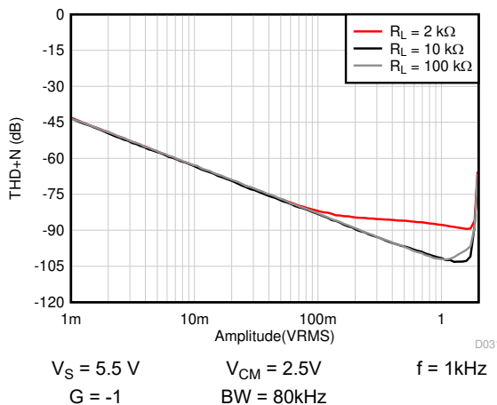
図 5-34. THD + N と振幅との関係
