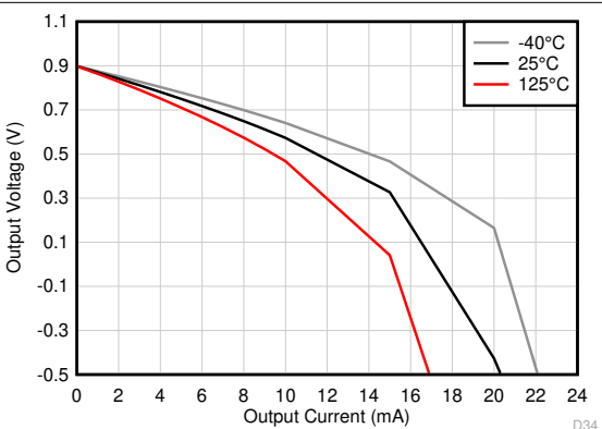
図 5-21. 出力電圧スイングと出力電流との関係 (ソース)
