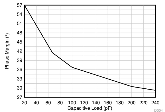
図 5-40. 位相マージンと容量性負荷との関係
