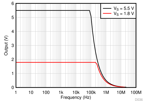
図 5-50. 最大出力電圧と周波数との関係
