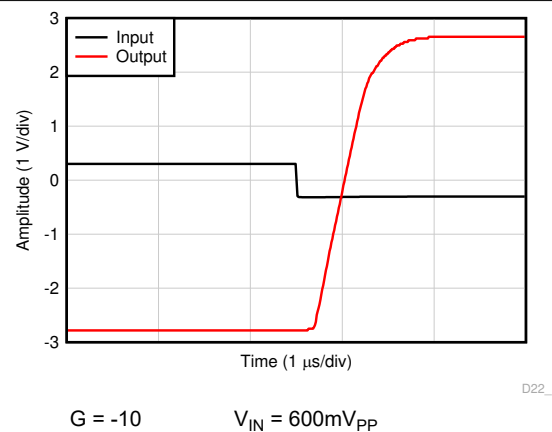
図 5-42. 過負荷回復
