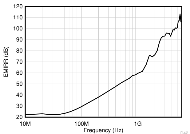
図 6-4. EMIRR テスト
