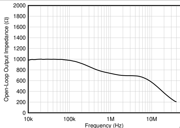
図 5-19. 開ループ出力インピーダンスと周波数との関係
