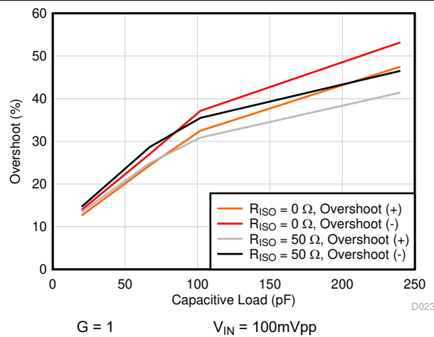
図 5-39. 小信号オーバーシュートと容量性負荷との関係
