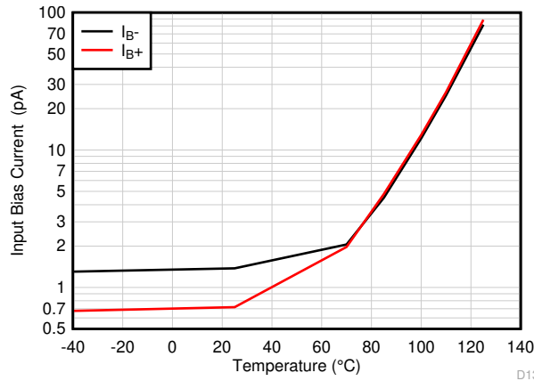
V_S = 5.5\text{V} , V_{CM} = V_S/2 図 5-13. I_B と温度との関係
