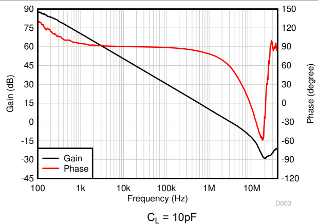
C_L = 10\text{pF} 図 5-18. 開ループゲインおよび位相と周波数との関係
