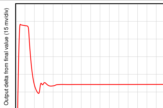
図 5-46. 大信号ステップ応答
