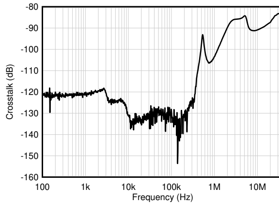
図 5-53. チャンネル セパレーション
