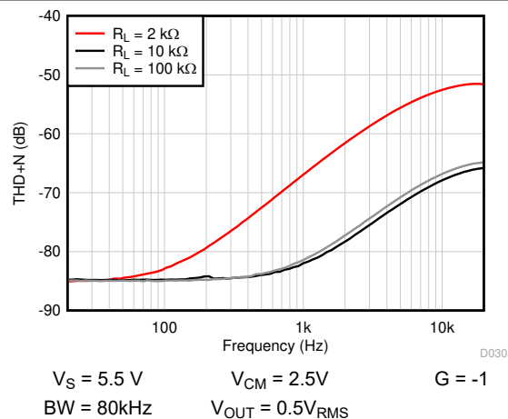
図 5-32. THD + N と周波数との関係
