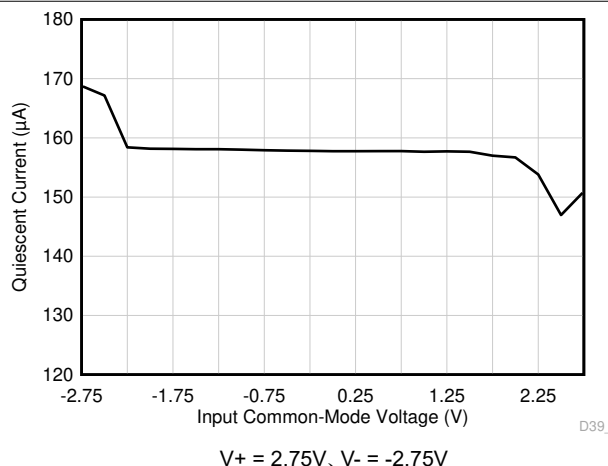
図 5-36. 静止電流と同相電圧との関係
