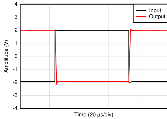
図 5-49. 大信号ステップ応答
