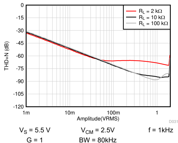
図 5-33. THD + N と振幅との関係
