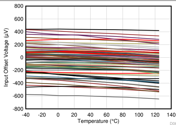
図 5-7. 入力オフセット電圧と温度との関係
