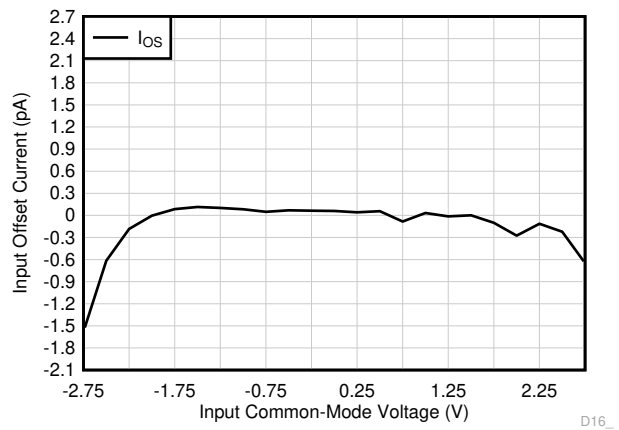
V_+ = 2.75\text{V} , V_- = -2.75\text{V} , V_{CM} = V_S/2 図 5-16. I_{OS} と同相電圧との関係
