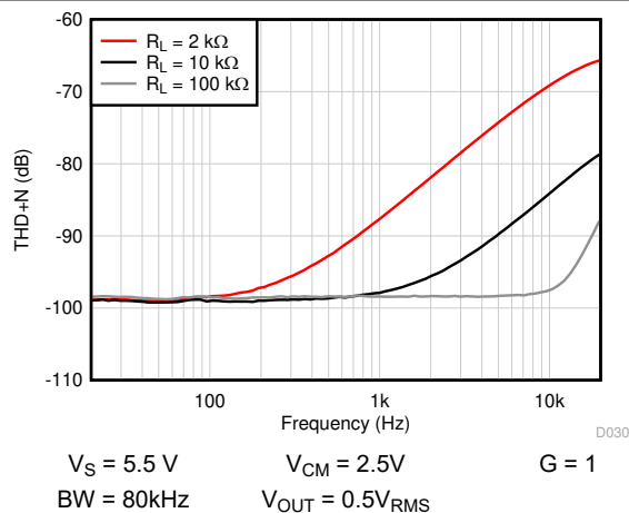
図 5-31. THD + N と周波数との関係
