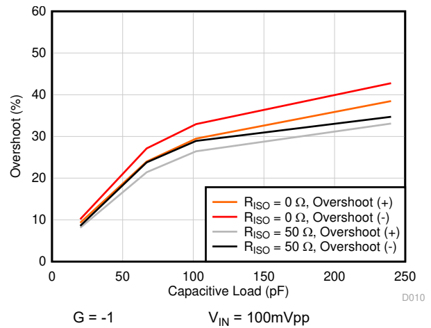
図 5-38. 小信号オーバーシュートと容量性負荷との関係
