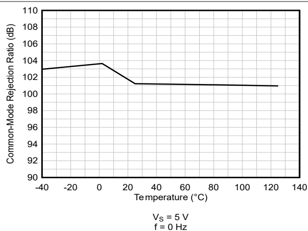
图 5-23. CMRR vs Temperature
