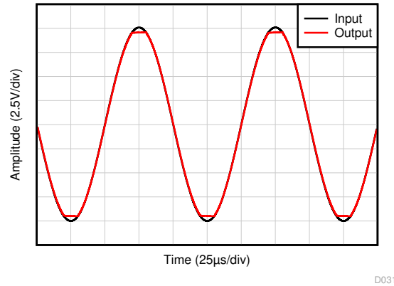
図 6-9. No Phase Reversal
