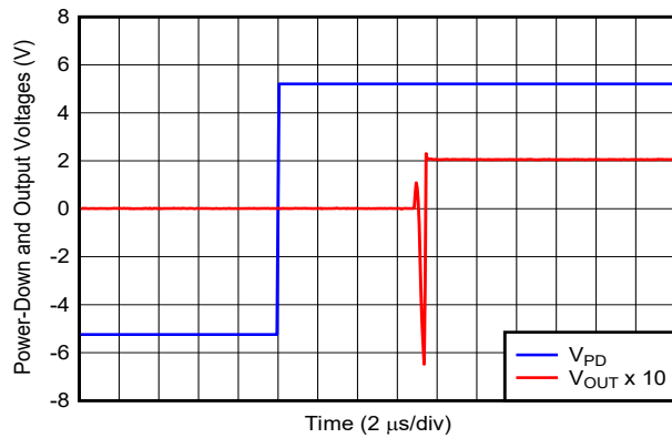
図 6-25. Turn-On Time to DC Input
