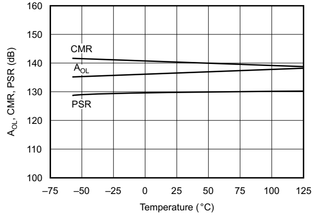
図 6-10. A_{OL} , CMR, PSR と温度との関係
