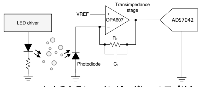
OPAx607 によるトランスインピーダンスのアプリケーション
