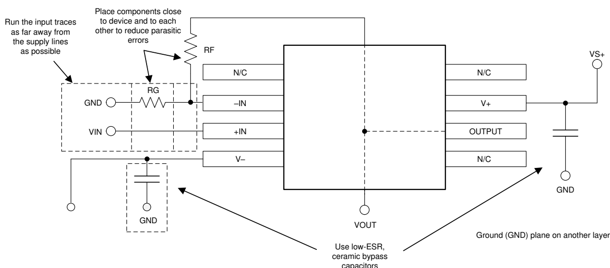
10-2. Layout Example
