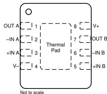
図 5-2. OPA2387 : D パッケージ、8 ピン SOIC および 図 5-3. OPA2387 : DSG パッケージ、8 ピン WSON (露出サーマル・パッド付き) (上面図) DGK パッケージ、8 ピン VSSOP
