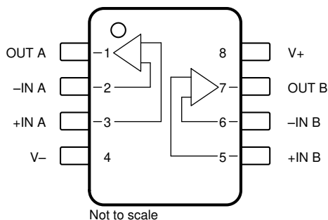
図 5-2. OPA2387 : D パッケージ、8 ピン SOIC および 図 5-3. OPA2387 : DSG パッケージ、8 ピン WSON (露出サーマル・パッド付き) (上面図) DGK パッケージ、8 ピン VSSOP
