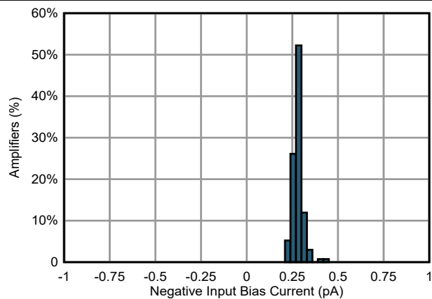
図 5-11. 負の入力バイアス電流の分布
