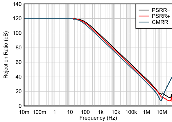
図 5-15. CMRR および PSRR と周波数との関係
