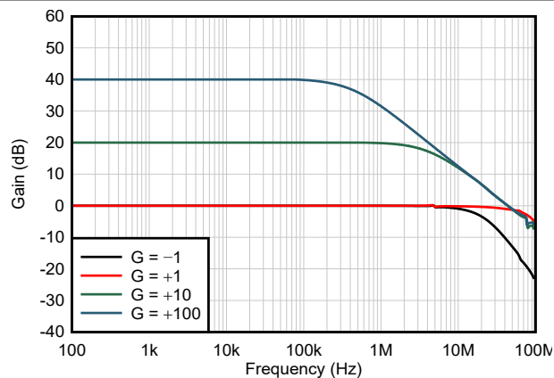
図 5-31. 開ループ・ゲインと周波数との関係
