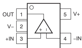
図 4-1. OPA328 DBV パッケージ、 5 ピン SOT-23 (上面図)
