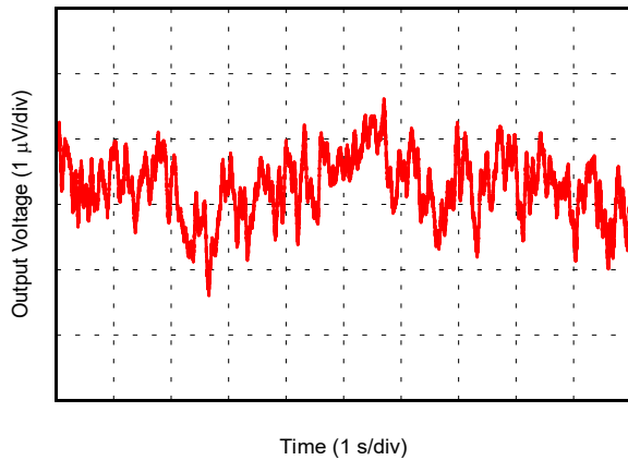
図 5-17. 0.1Hz~10Hz の入力電圧ノイズ
