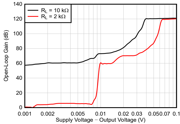
図 5-25. 開ループ・ゲインと電源電圧デルタへの出力との関係
