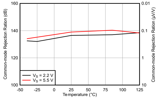
図 5-14. CMRR と温度との関係
