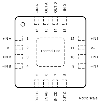
図 4-7. OPA4328 RUM パッケージ (開発中製品)、16 ピン WQFN (上面図)
