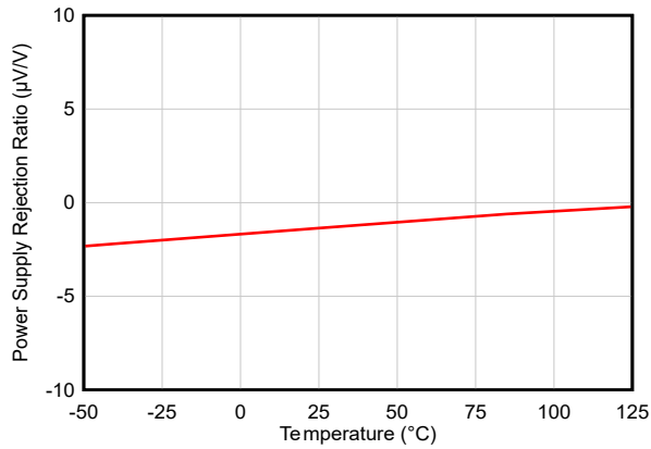
図 5-13. PSRR と温度との関係
