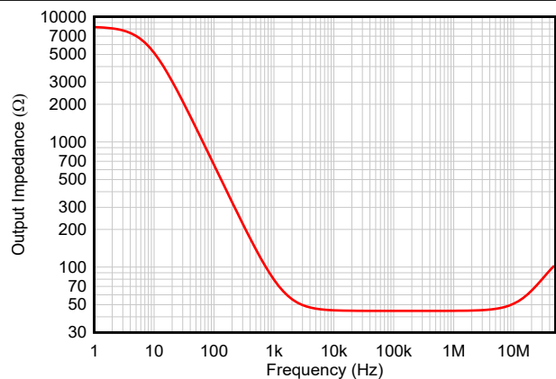
図 5-24. 開ループの出力インピーダンスと周波数との関係
