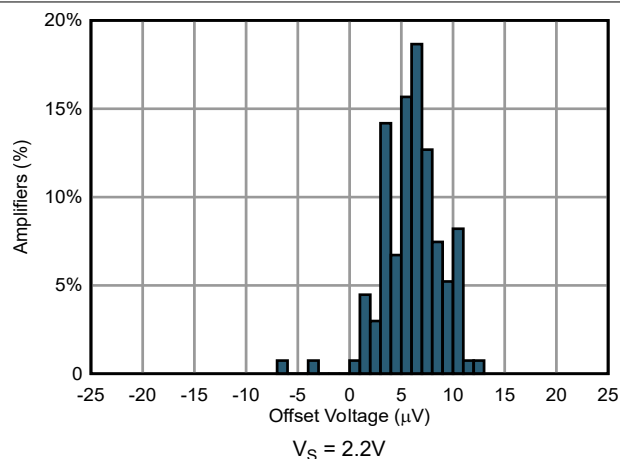
図 5-1. オフセット電圧の製品分布
