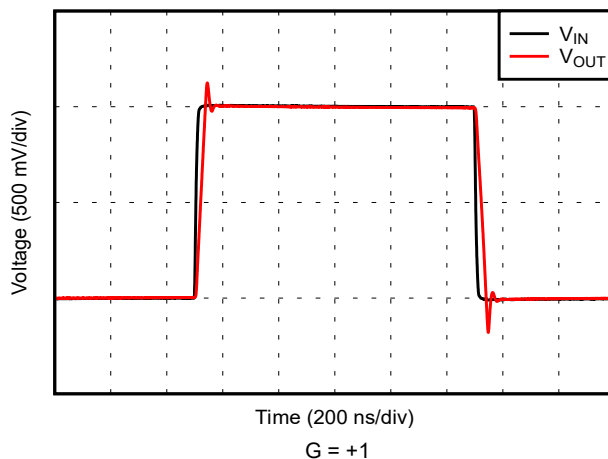
図 5-35. 大信号ステップ応答
