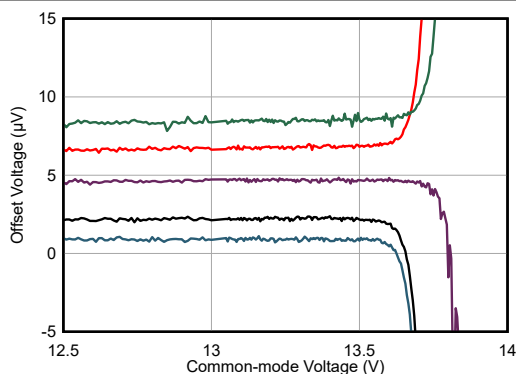
図 5-13. High 電源でのオフセット電圧と V_{CM} との関係
