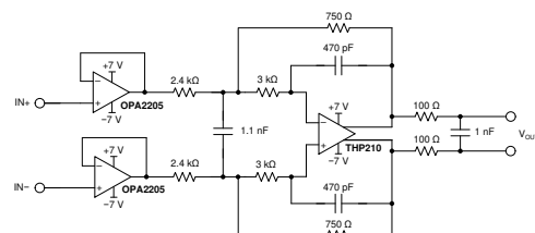
OPA2205 の代表的なアプリケーション
