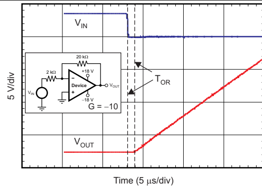
FIG 26. No Phase Reversal
