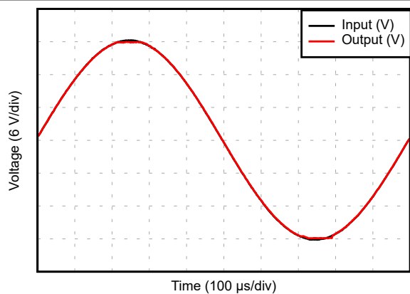
図 5-32. 位相反転なし
