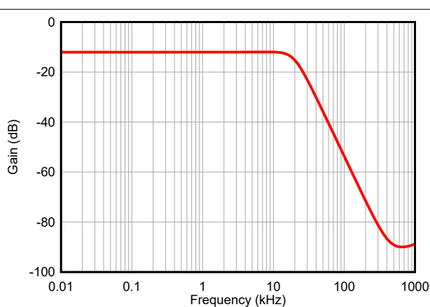
図 8-3. アッテネータ + フィルタ応答
