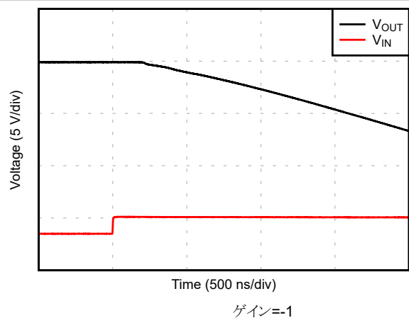
図 5-36. 正の過負荷からの回復
