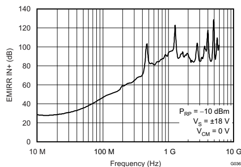
EMIRR IN+と周波数との関係
