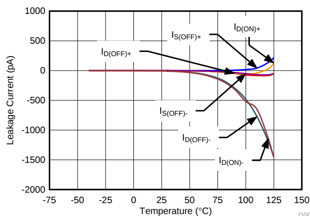
リーク電流と温度
