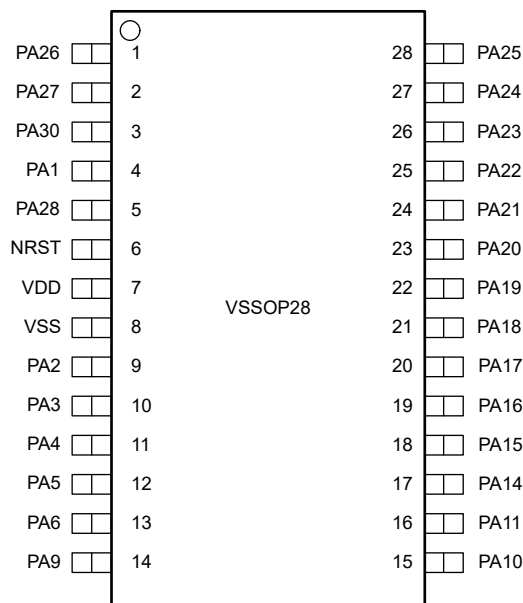
図 6-7. 28 ピン DGS28 (VSSOP) (上面図)
