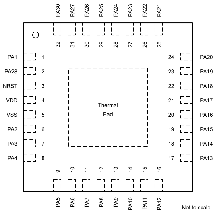
図 6-5. 32 ピン RHB (VQFN) (上面図)
