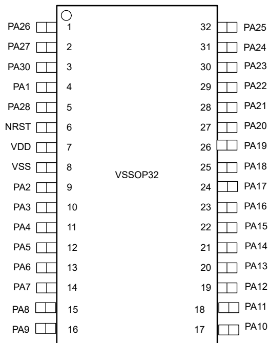
図 6-6. 32 ピン DGS32 (VSSOP) (上面図)
