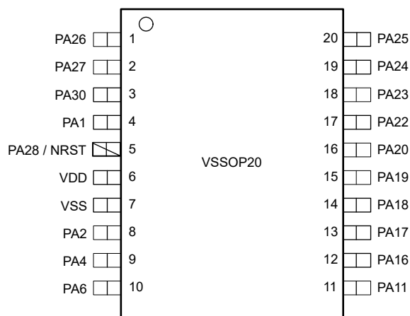
図 6-9. 20 ピン DGS20 (VSSOP) (上面図)
