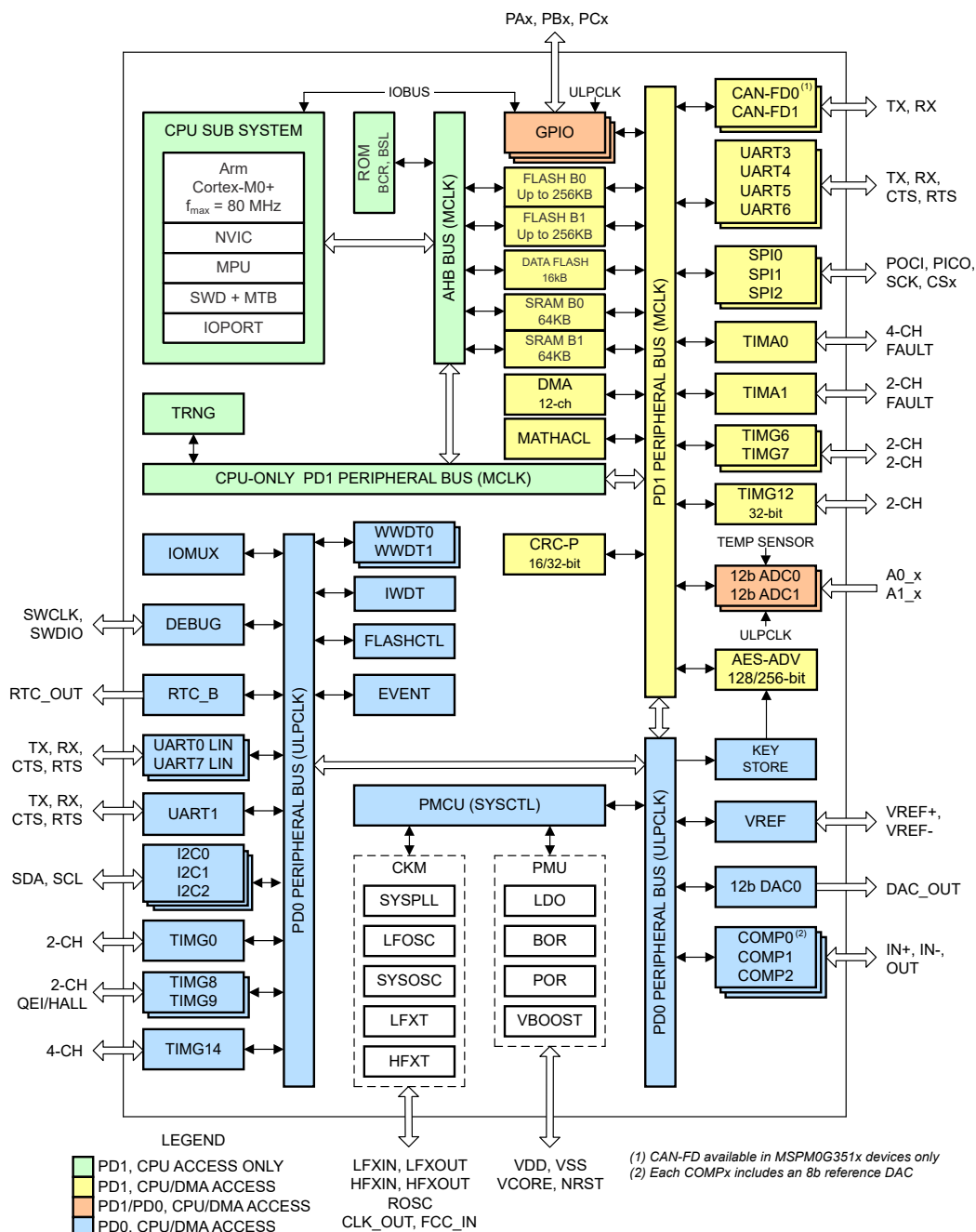
図 8-1. MSPM0G352x-Q1 の機能ブロック図
