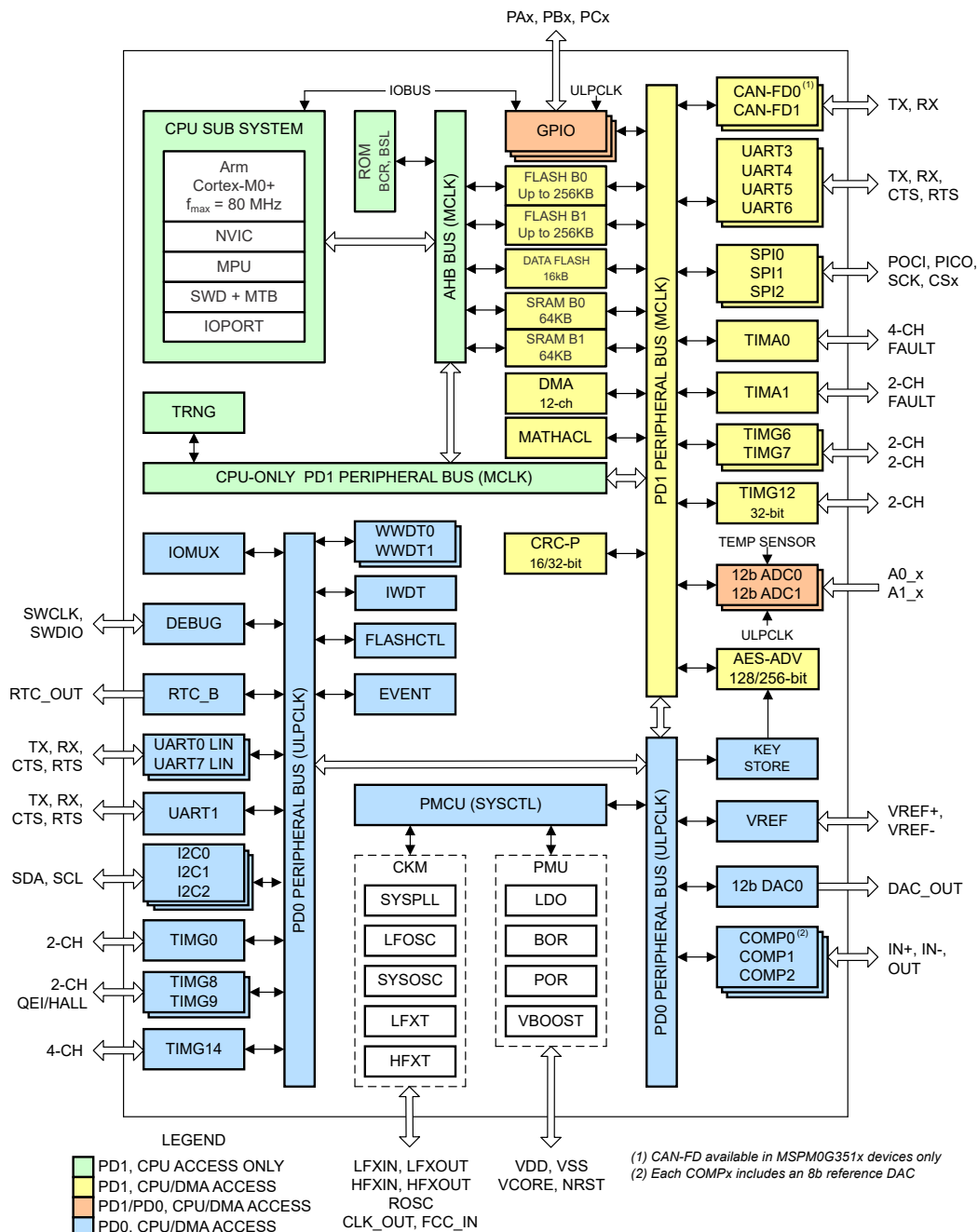
図 4-1. MSPM0G352x-Q1 の機能ブロック図
