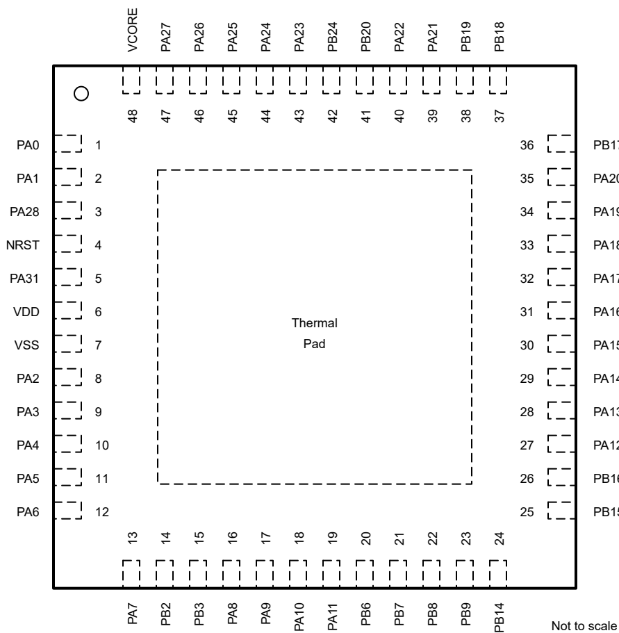
図 6-5. 48 ピン RGZ (0.5mm) (VQFN) パッケージ図
