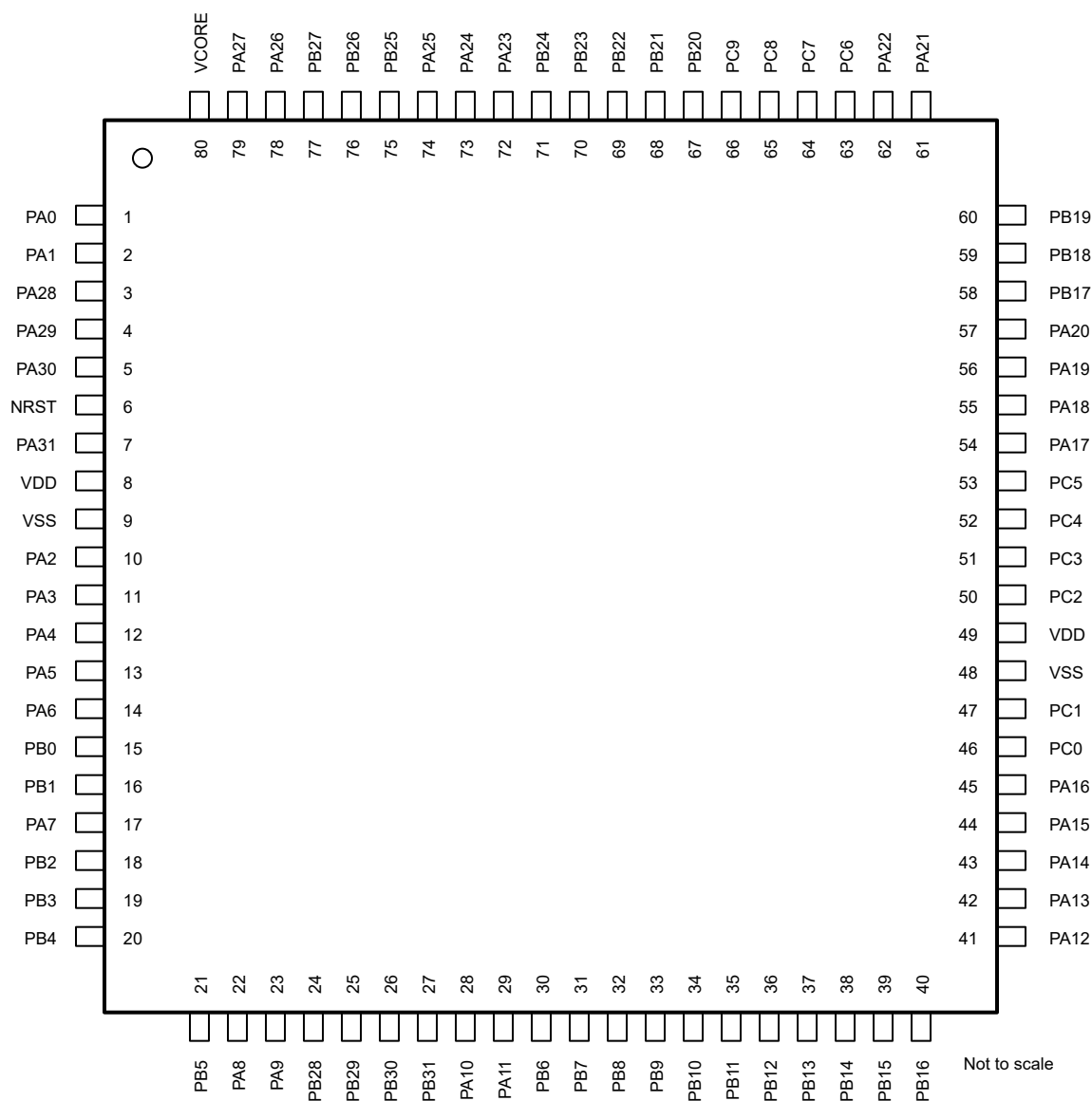
図 6-2. 80 ピン PN (0.5mm) (LQFP) パッケージ図
