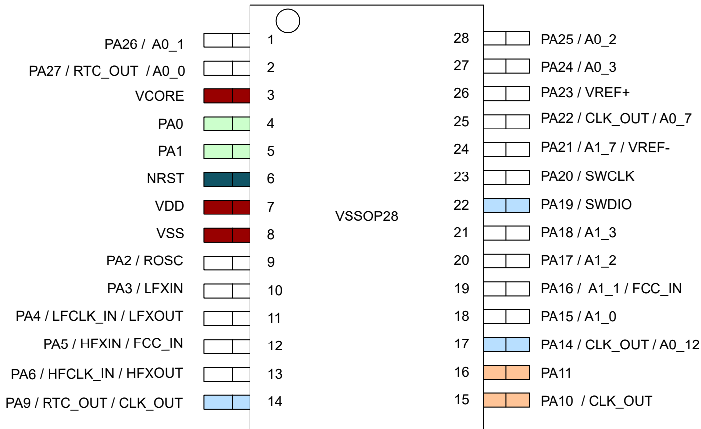
図 6-6. 28 ピン DGS28 (VSSOP) (上面図)
