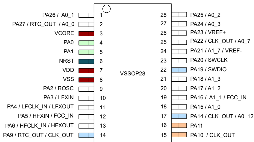
図 6-7. 28 ピン DGS28 (VSSOP) (上面図)
