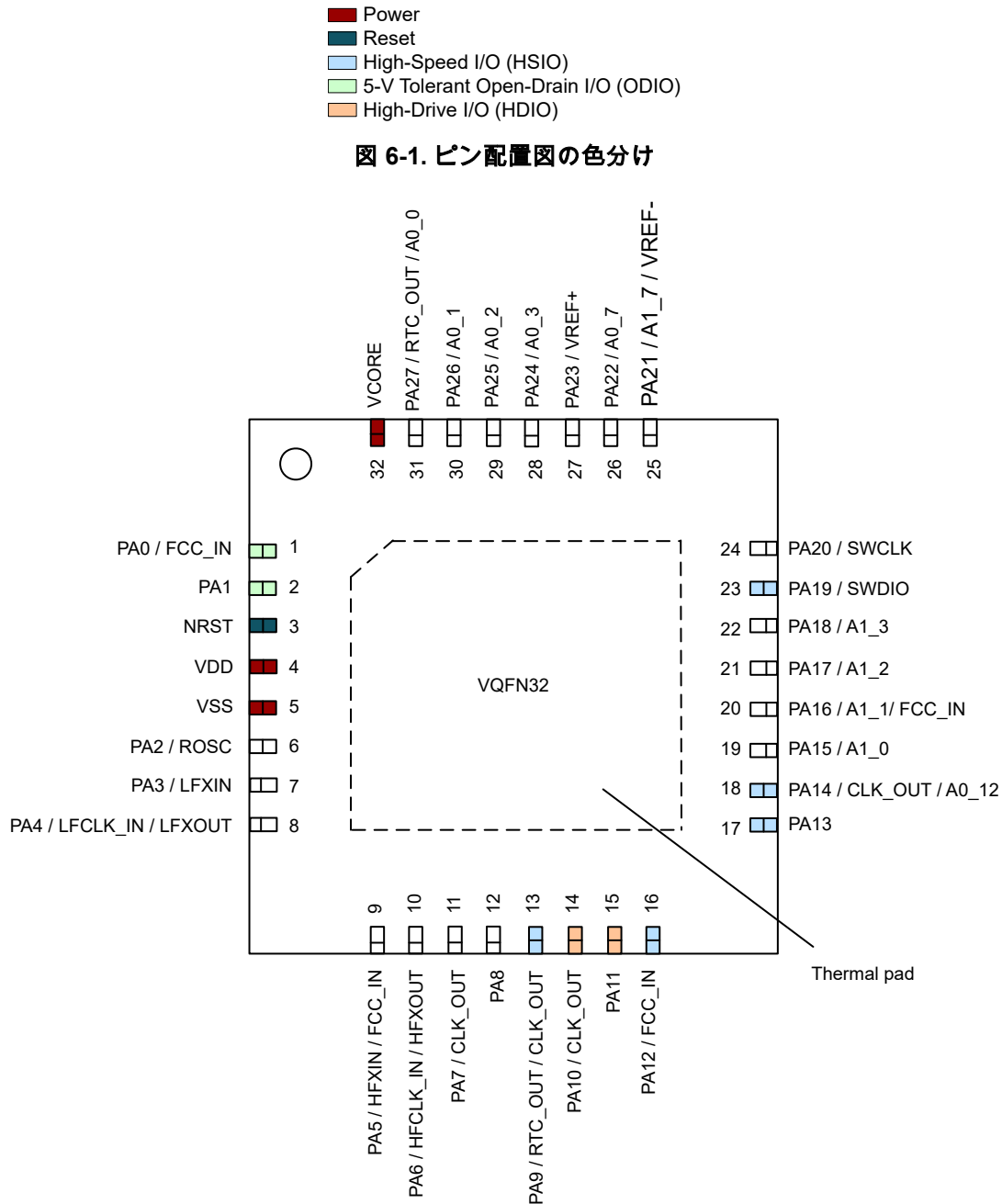
図 6-2. 32 ピン RHB (VQFN) (上面図)
