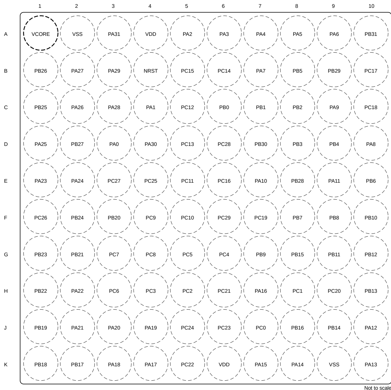
図 6-1. 100 ピン Zow (0.8mm) (nFBGA)パッケージ図
