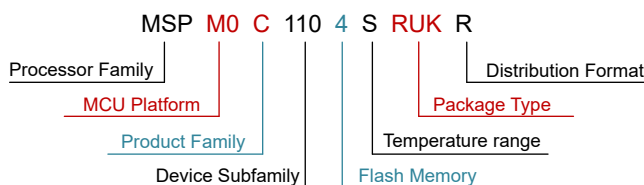
図 10-1. Device Nomenclature
