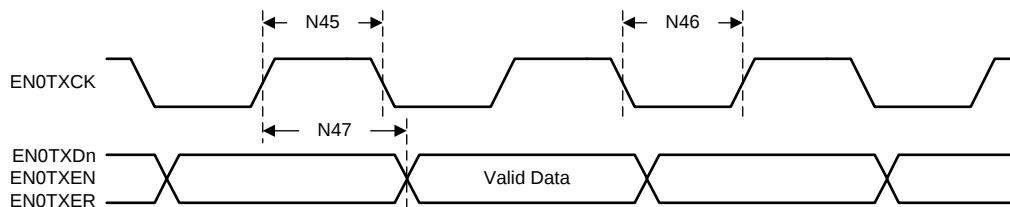
图 5-40. 10-Mbps MII Transmit Timing
