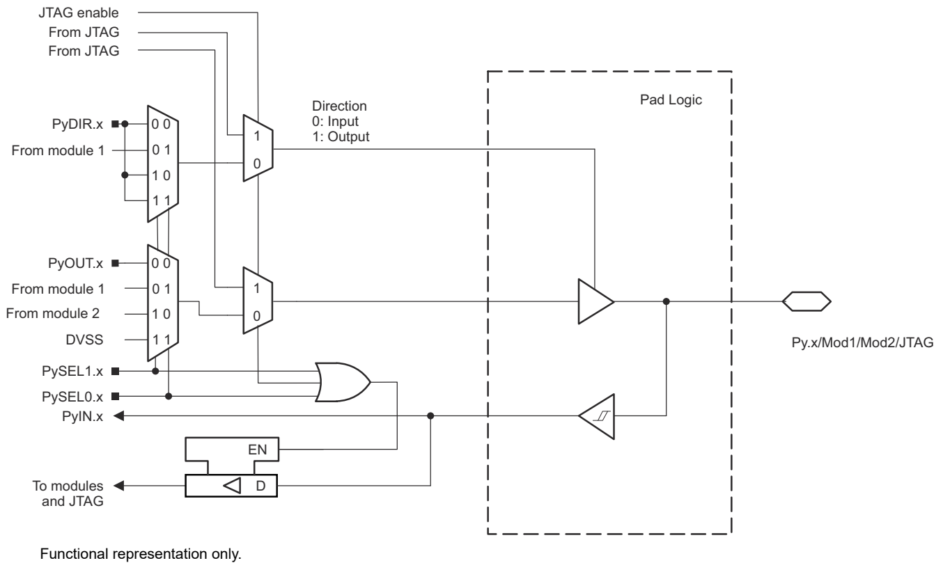
図 9-8. Py.x/Mod1/Mod2/JTAG Pin Diagram
