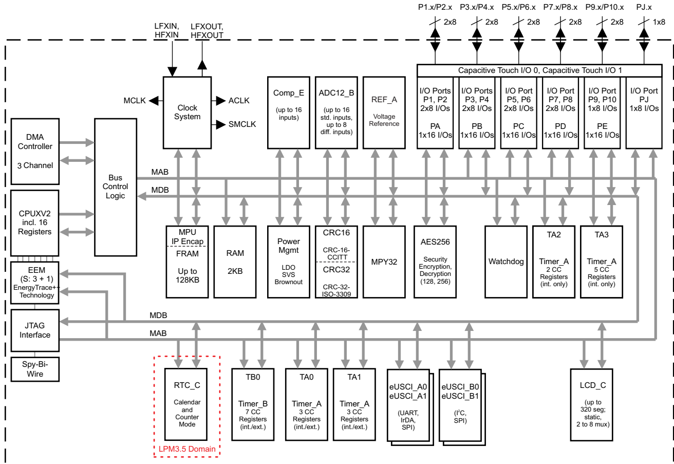
図 1-1. 機能ブロック図 – MSP430FR697x、MSP430FR697x1
