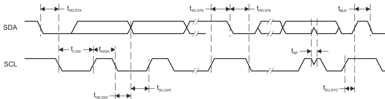
图 8-14. I 2 C 模式时序
