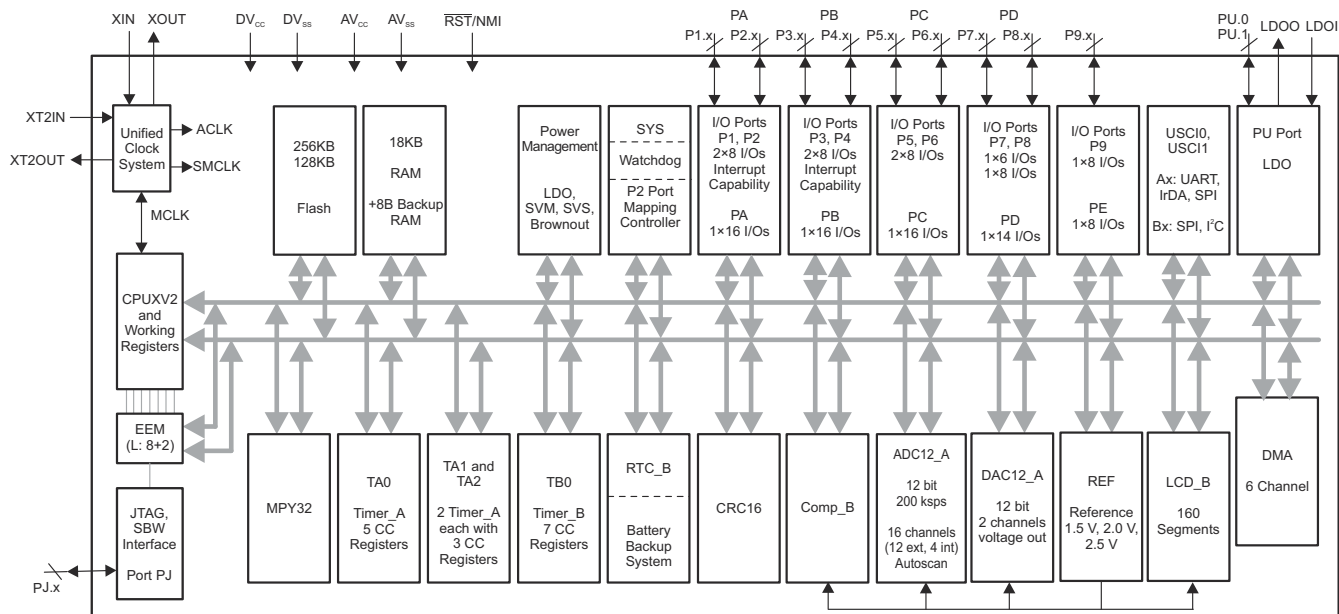
図 4-1. 機能ブロック図 – MSP430F6438, MSP430F6436
