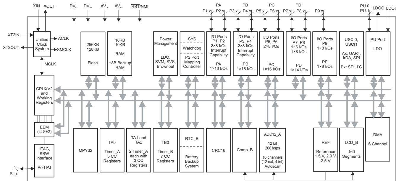
図 4-2. 機能ブロック図 – MSP430F6435, MSP430F6433
