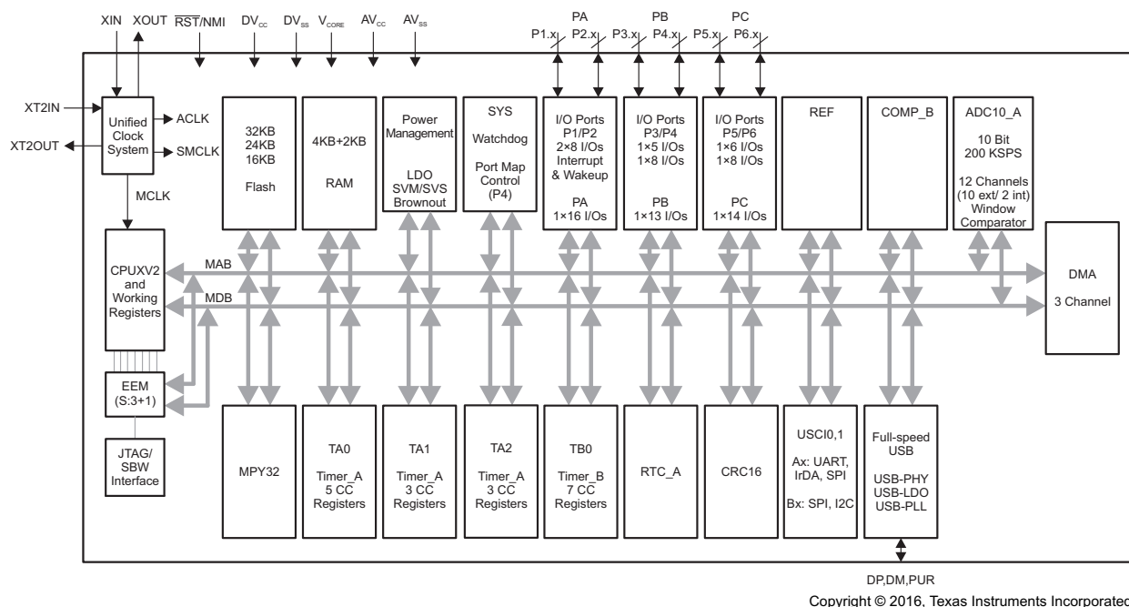
図 1-1. 機能ブロック図 – MSP430F5510IRGC、MSP430F5509IRGC、MSP430F5508IRGC、MSP430F5510IZQE、MSP430F5509IZQE、MSP430F5508IZQE
