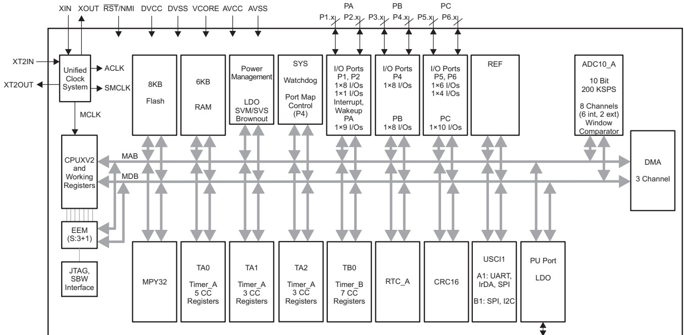
図 1-2. 機能ブロック図 - MSP430F5310IRGZ、MSP430F5309IRGZ、MSP430F5308IRGZ、MSP430F5310IPT、MSP430F5309IPT、MSP430F5308IPT
