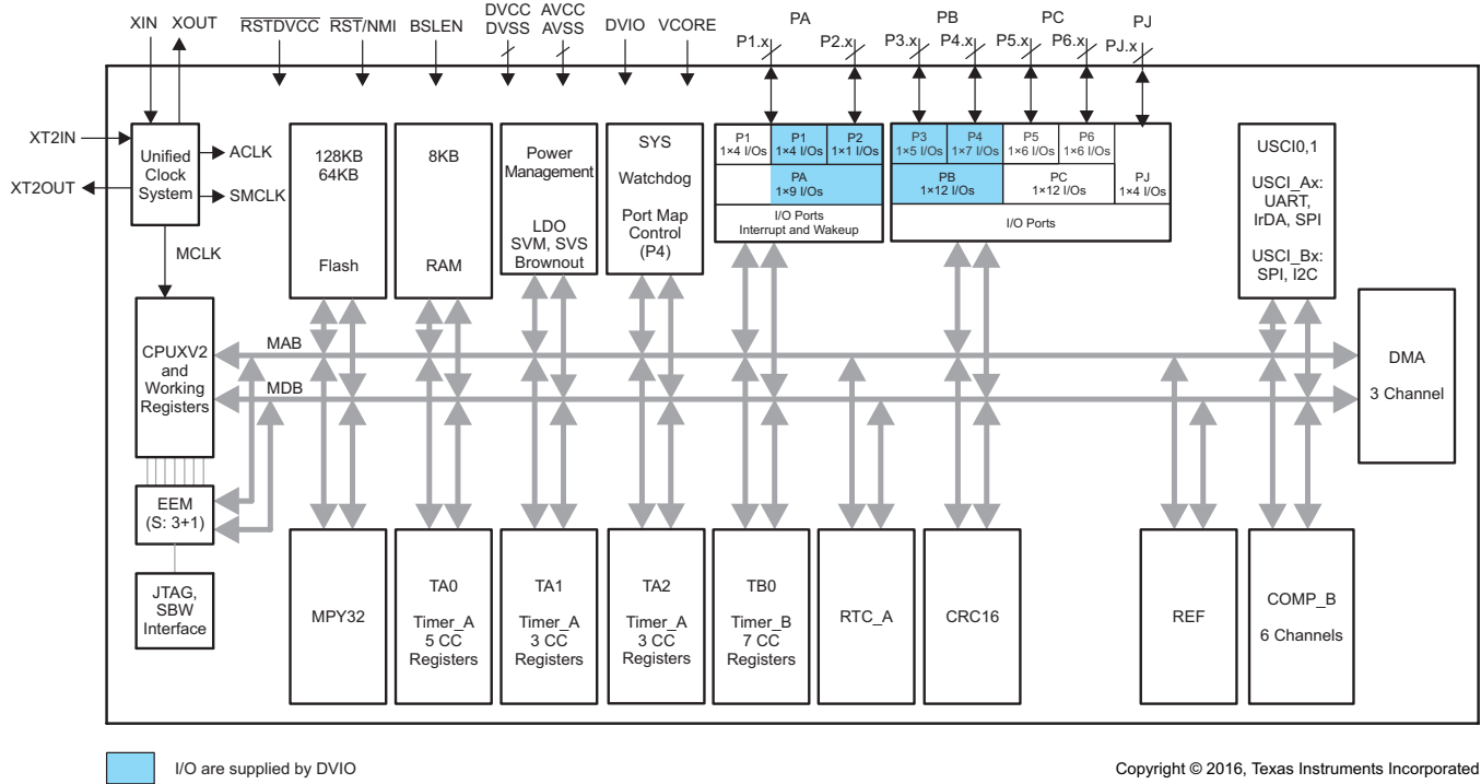
図 1-4. 機能ブロック図 – F5214、F5212 – RGZパッケージ
